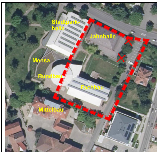
Abb. 2: Abgrenzung des Vorhabengebietes innerhalb des Bebauungsplans „Östlicher Promenadenweg, 2. Änderung“. Zwei der hier noch im Luftbild dargestellten drei Bäume (Robinien, s. kleines Foto) wurden im Winter 2021/2022 gefällt (rotes Kreuz).
