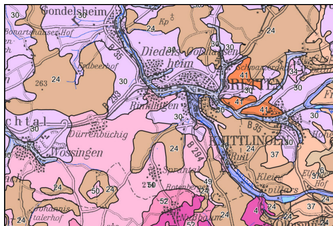
Abb. 10: Böden im Plangebiet
