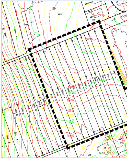
Abb. 9: Höhenlage und Relief
